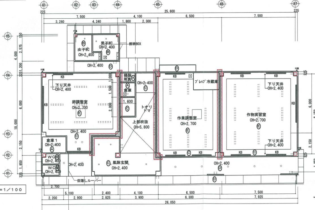
2階天井伏図 S=1/100
